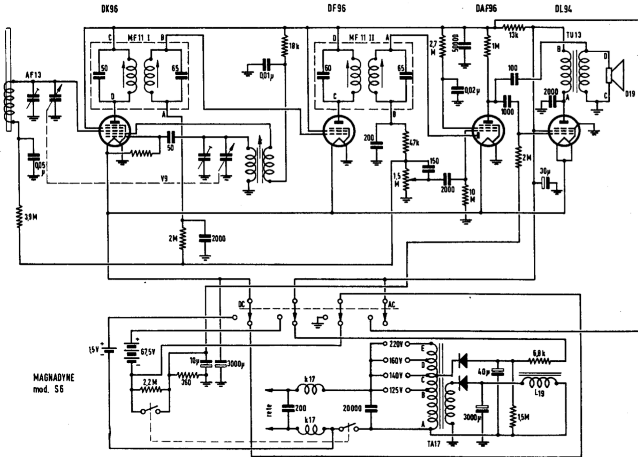
SCHEMA ELETTRICO DEL RADIORICEVITORE MAGNADYNE, MOD. S6
